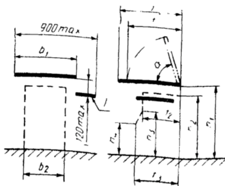
1—полка для чертежных и рисовальных принадлежностей
