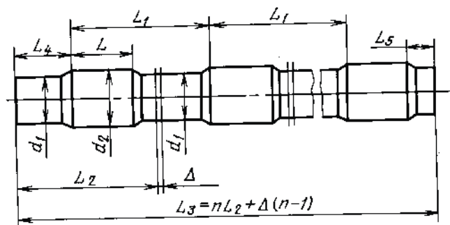
Размеры, мм
