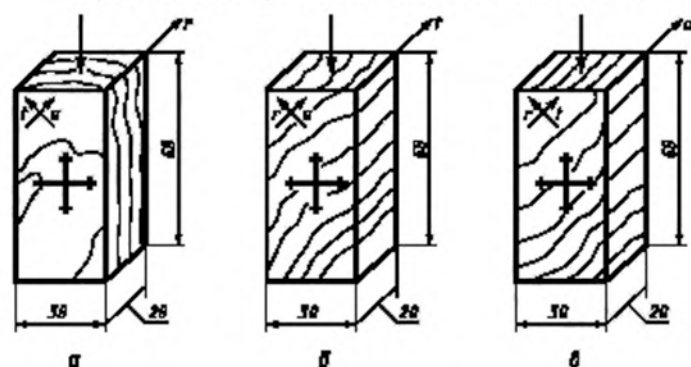
Форма и размеры образцов для определения модулей сдвига
