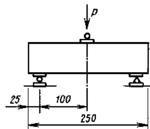
Схема испытания кирпича на изгиб
