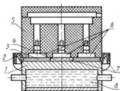
Схема электродного устройства
