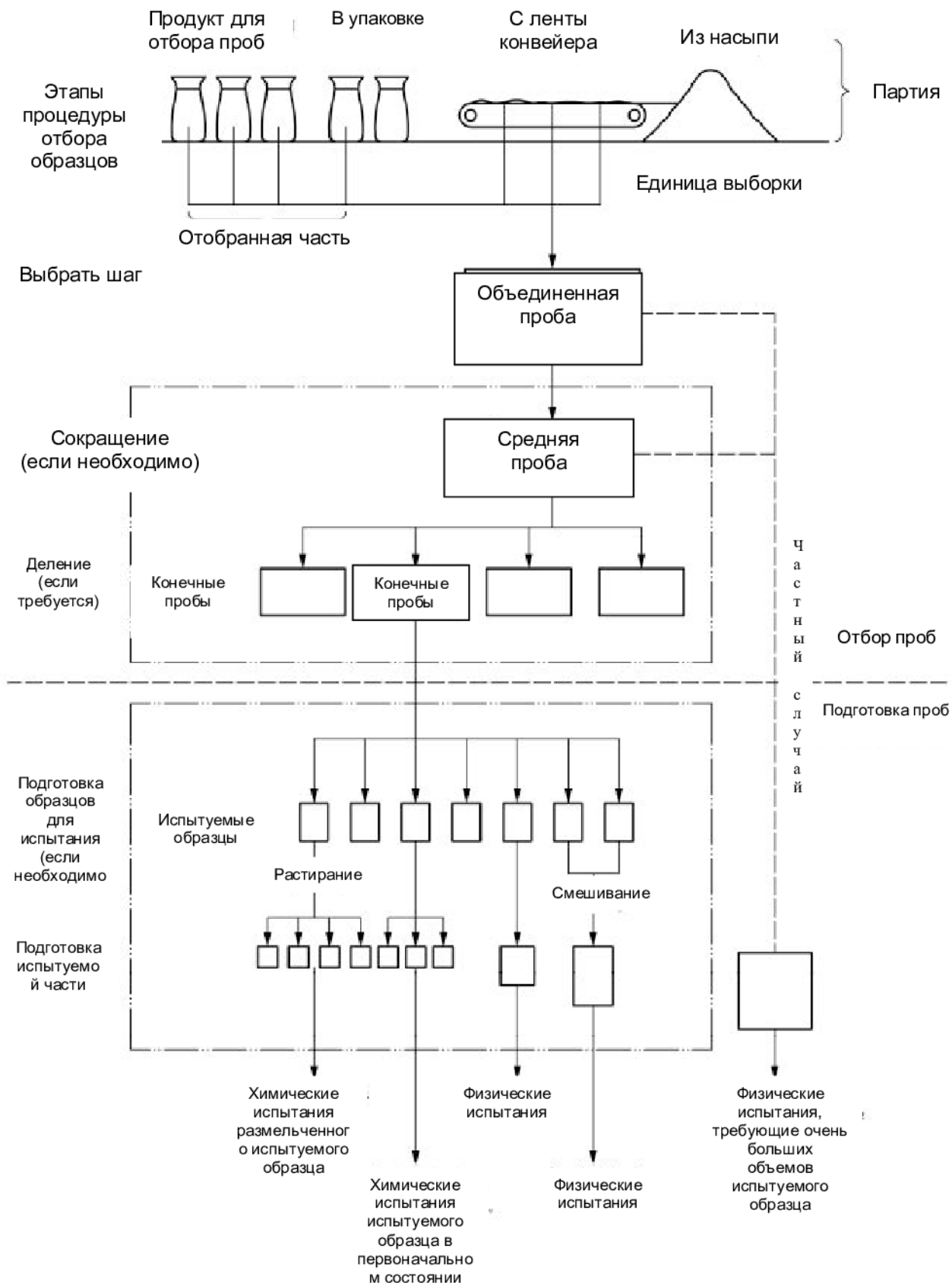
Рисунок 1 —Схема отбора проб твердых веществ
